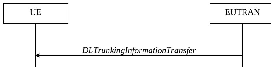
图12 集群下行直传
