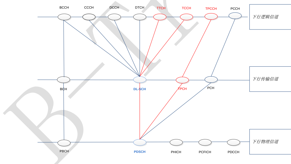
图 2 下行逻辑信道映射关系图
