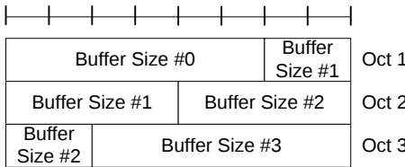
图 5 集群短 BSR 和集群削减 BSR MAC 控制单元
