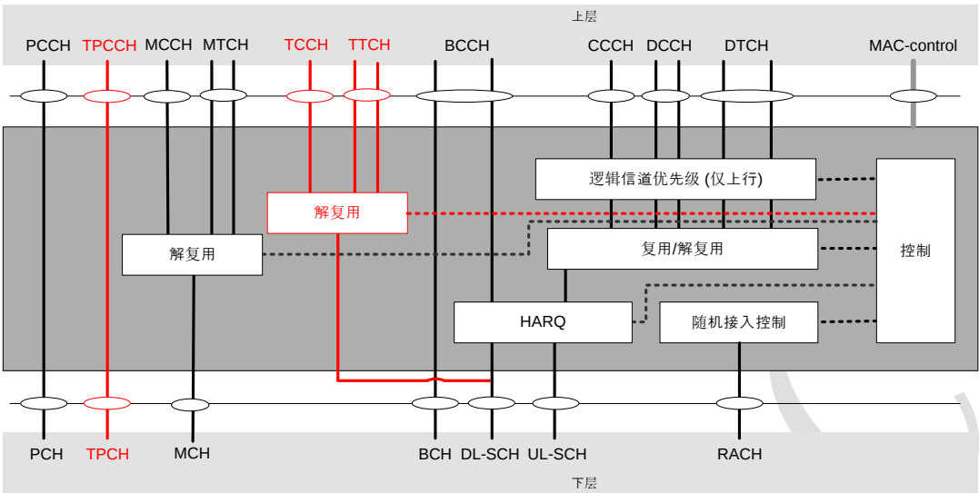
图 1 UE 侧 MAC 结构
