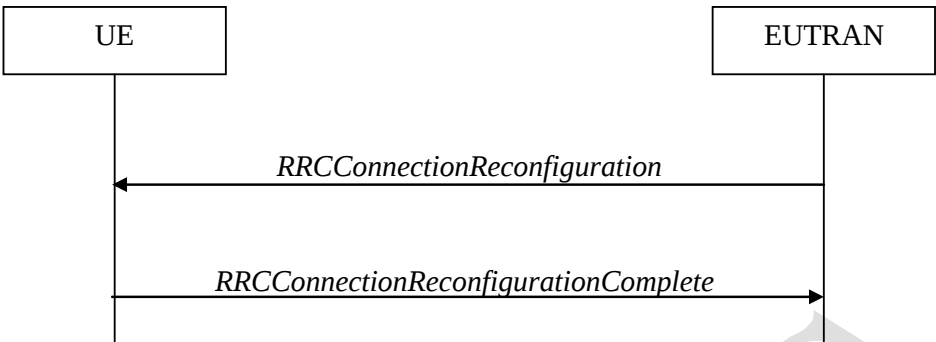
图10 RRC连接重配置
