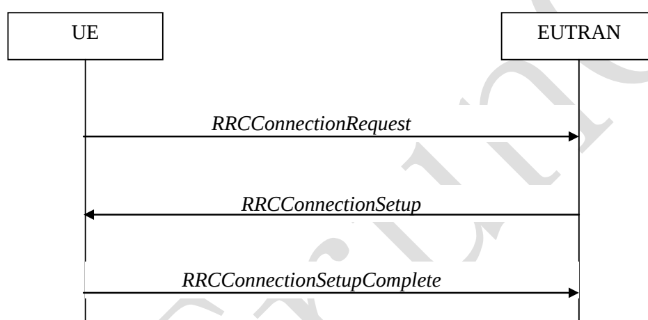
图9 RRC连接建立
